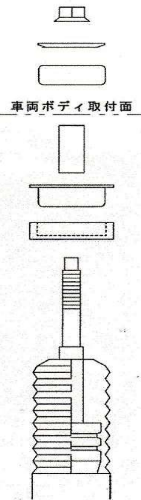
⑤ 純正ゴムブッシュ装着図
