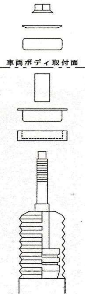
⑤ 純正ゴムブッシュ装着図
